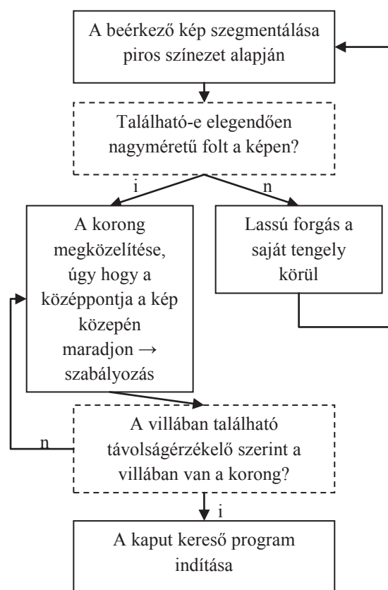
4. ábra. A korong keresésének blokk diagramja
