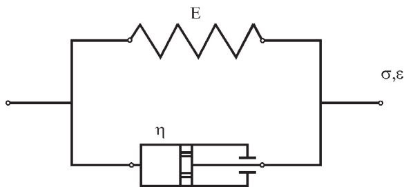
1. ábra: Az ékszíj mechanikai modellje
