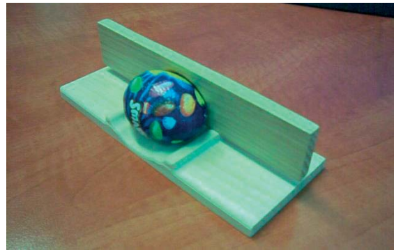
21. ábra. Gőzölt bükk anyagból készített feladó és betoló szerszámok a becsomagolt csokoládétojással együtt
