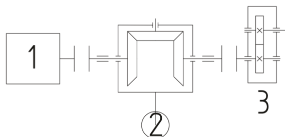
7. ábra. A mérés elve
