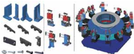
4. ábra. Moduláris felépítésű célgép elemei és alkalmazásuk
