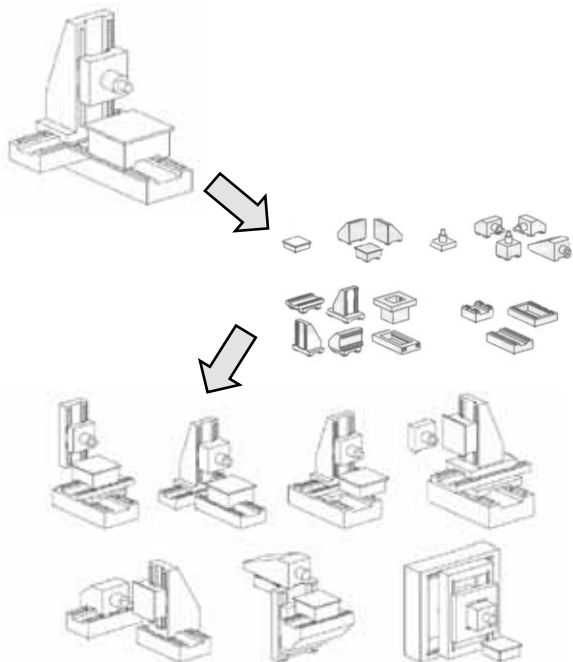
3. ábra. Moduláris szerszámgép alapgép, szerszámgép-elemek és néhány kombináció kialakítása
