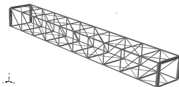
2. ábra. Rácsos hídszerkezet geometriai modellje.
